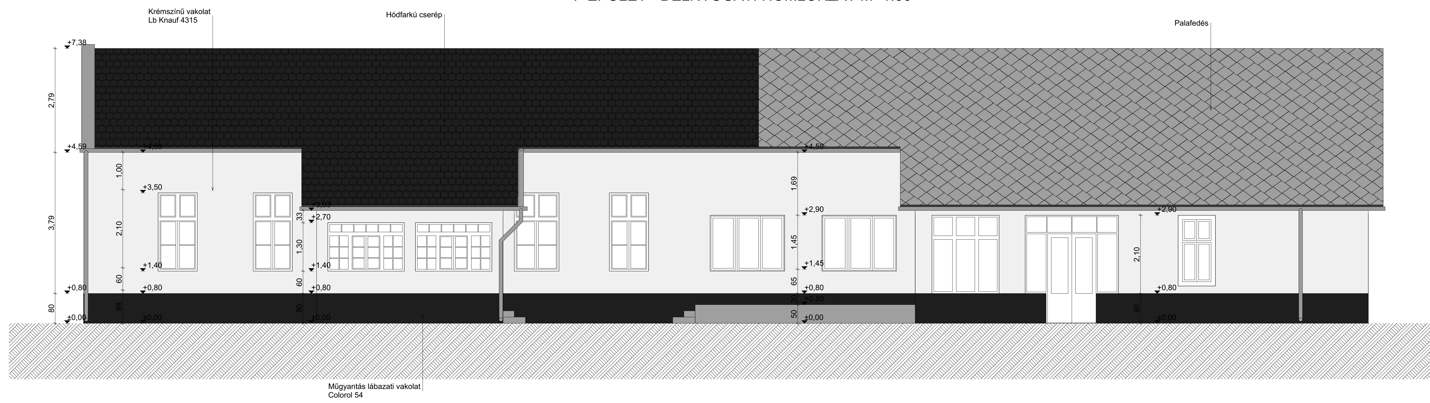
F ÉPÜLET - DÉLNYUGATI HOMLOKZAT M=1:50
