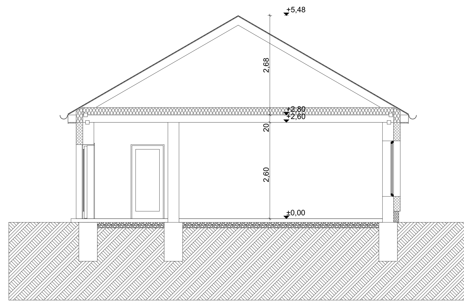
E METSZET M=1:50
