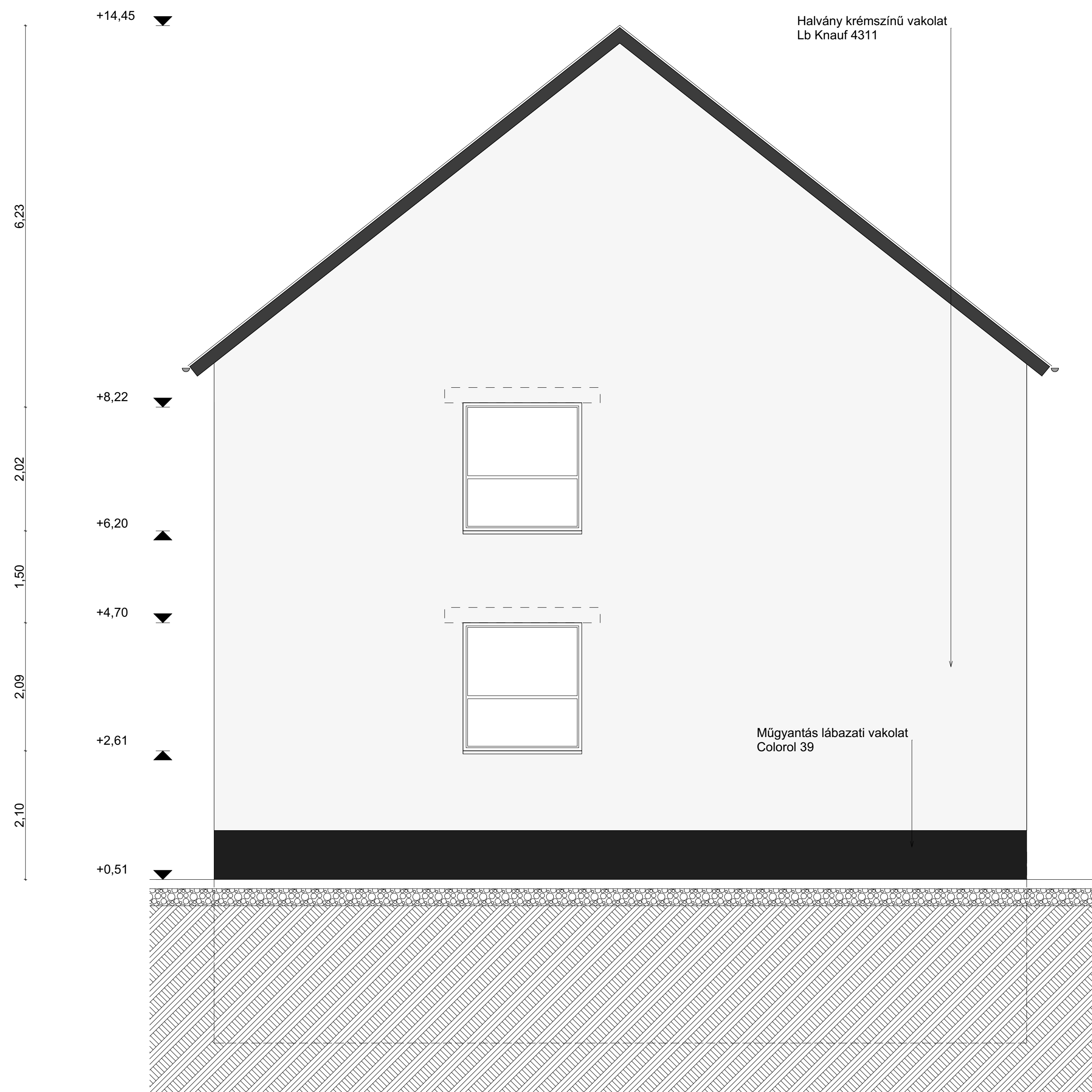
C ÉPÜLET - ÉSZAKNYUGATI HOMLOKZAT M=1:50
