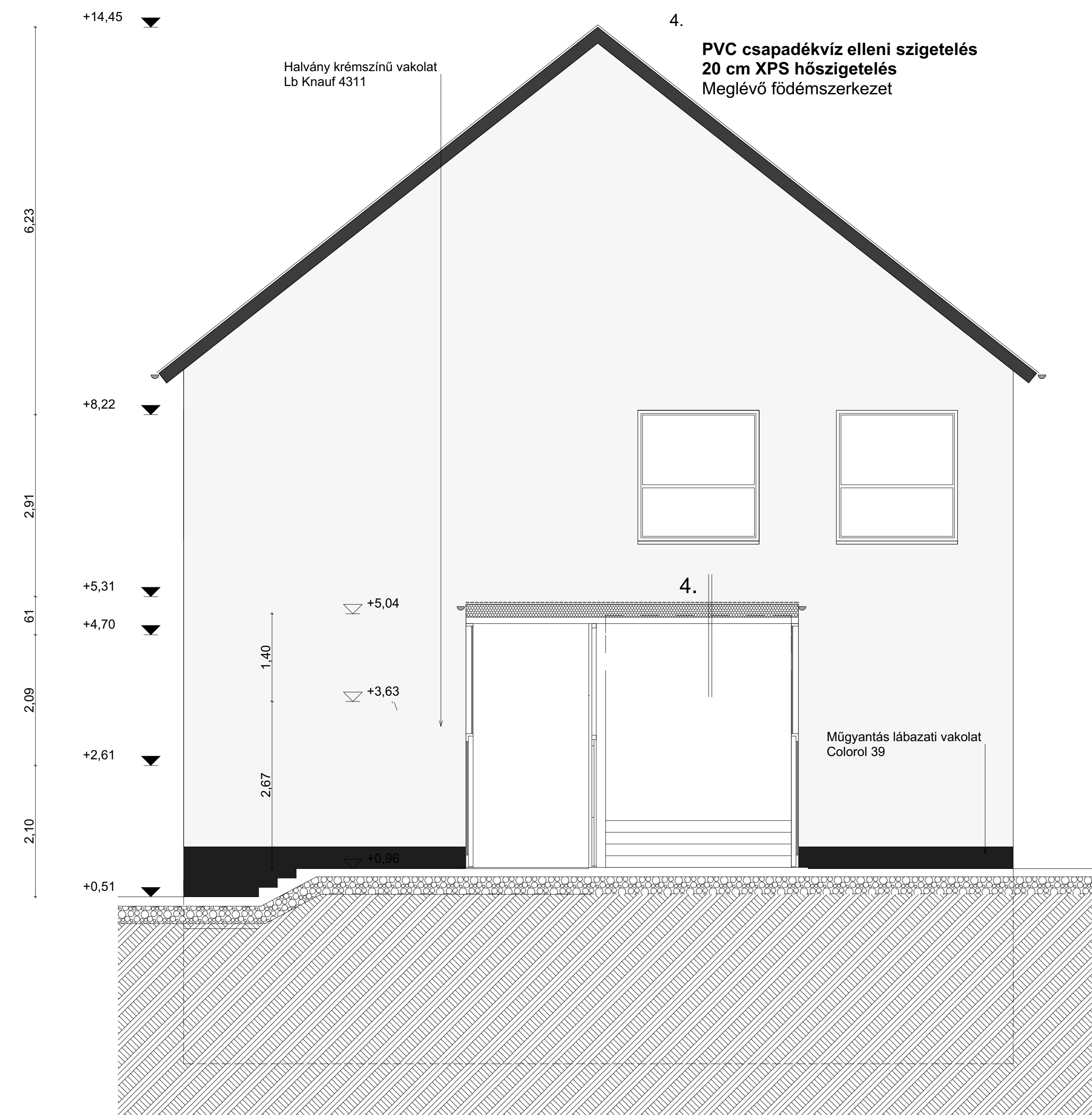
C3 - C3 METSZET M=1:50
