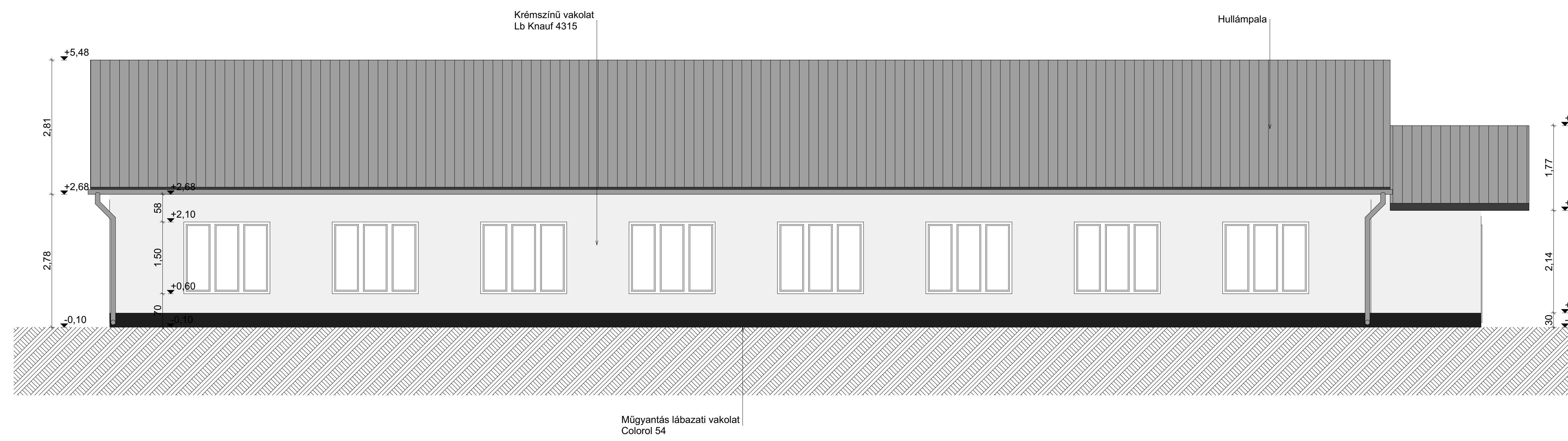
E ÉPÜLET - DÉLNYUGATI HOMLOKZAT M=1:50
