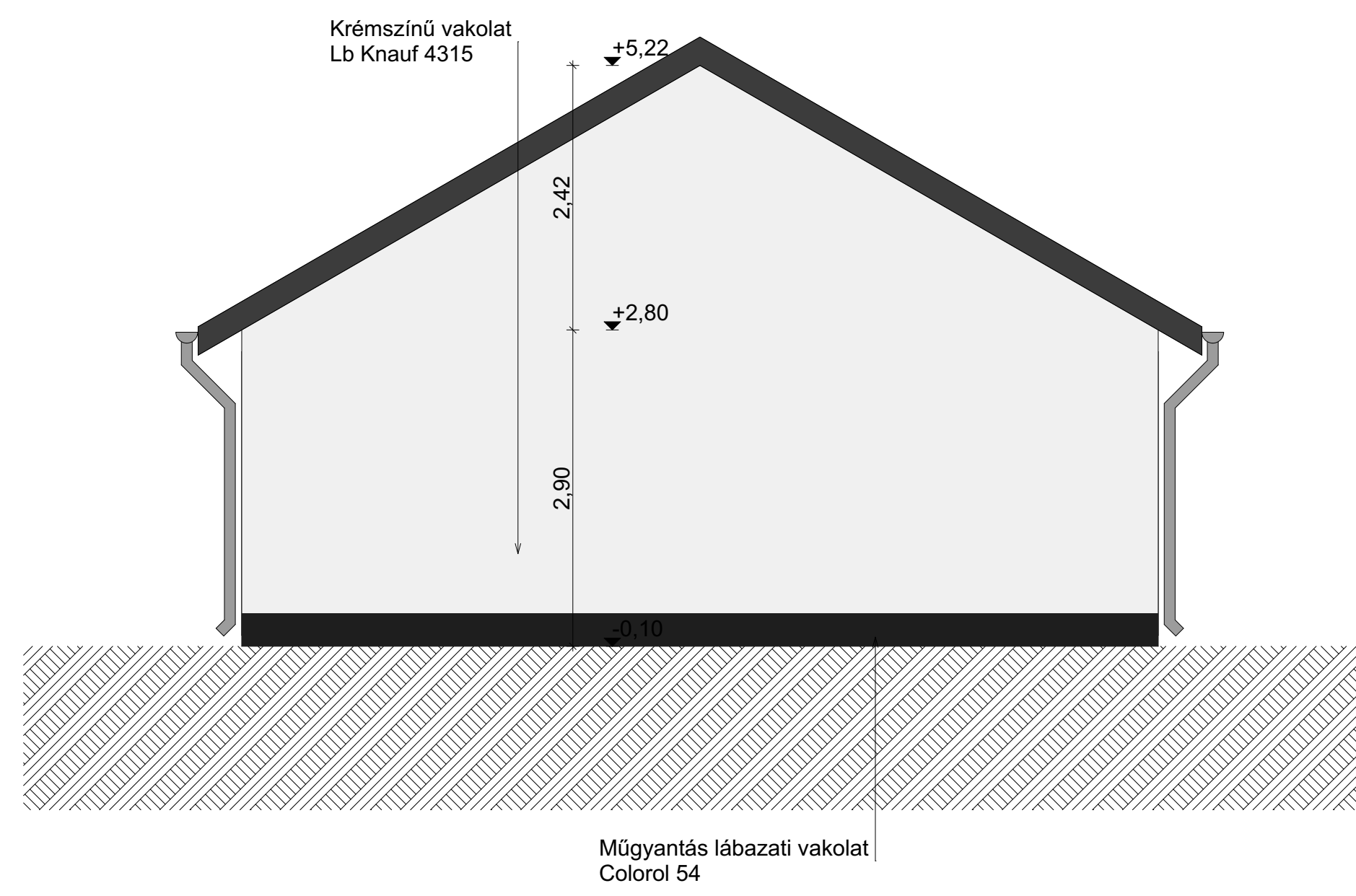
E ÉPÜLET - ÉSZAKNYUGATI HOMLOKZAT M=1:50
