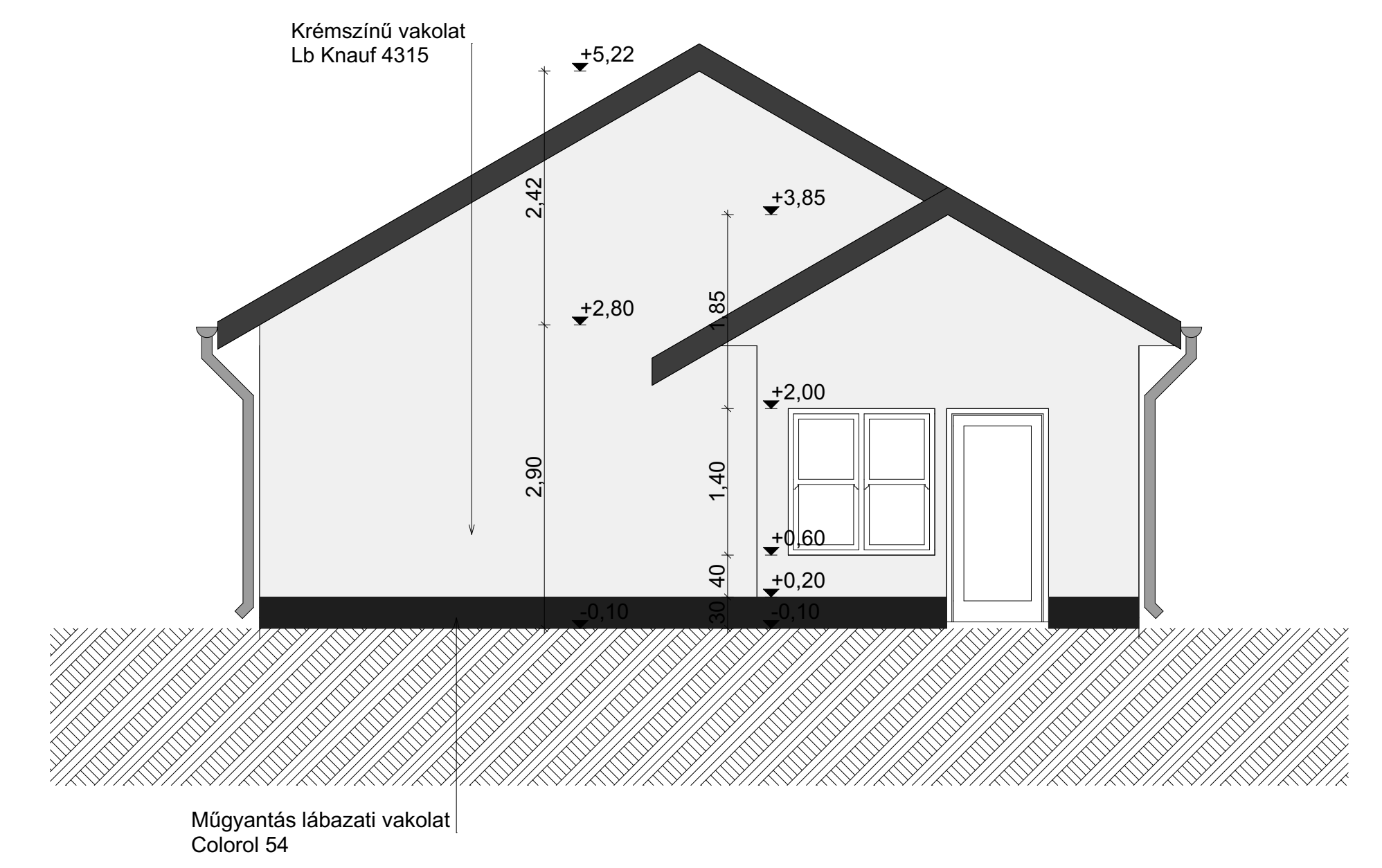
E ÉPÜLET - DÉLNYUGATI HOMLOKZAT M=1:50
