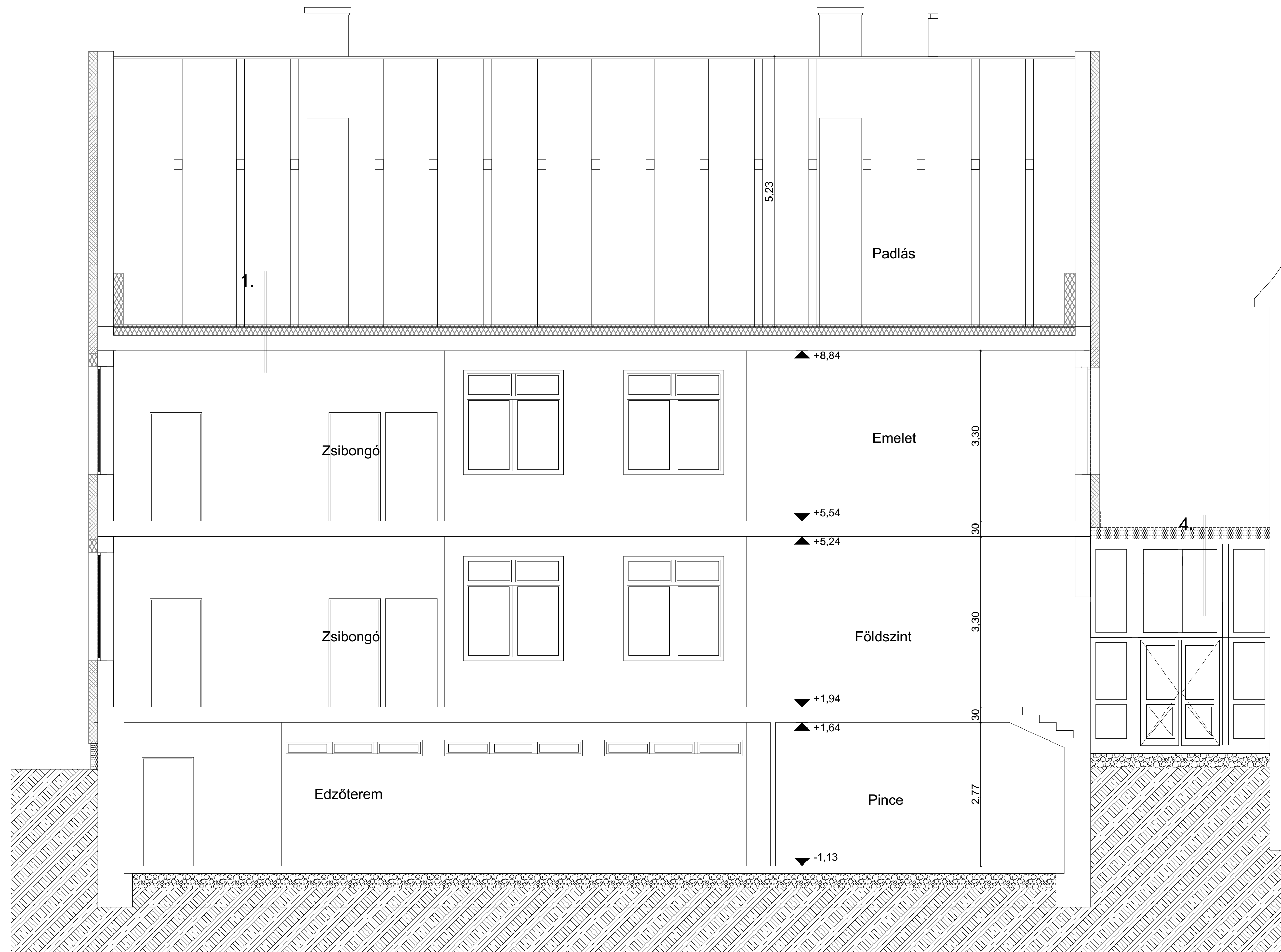
C1 - C1 METSZET M=1:50
