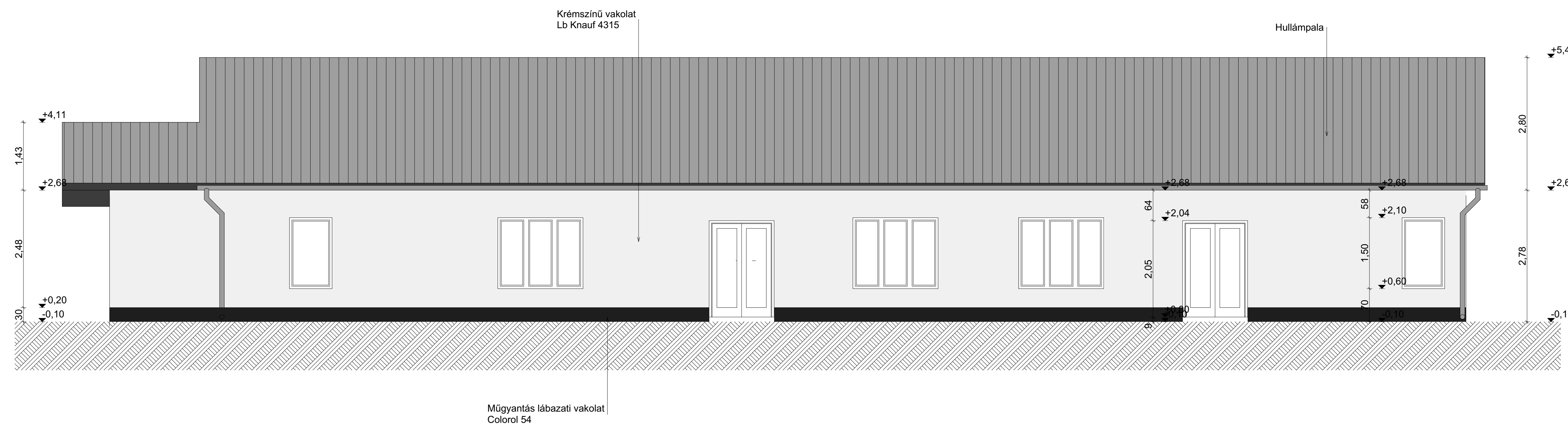
E ÉPÜLET - ÉSZAKKELETI HOMLOKZAT M=1:50
