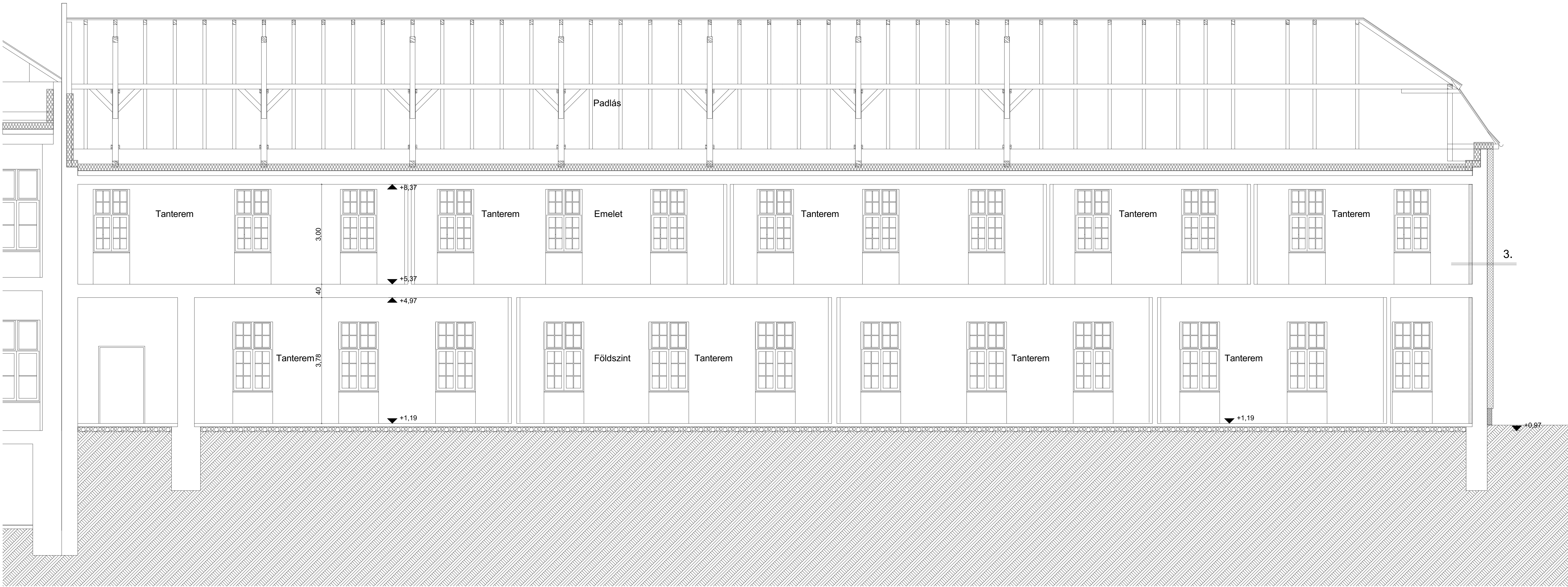
B3 - B3 METSZET M=1:50
