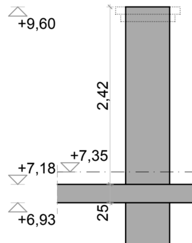
O2 OSZLOP NÉZETE KÉSZÜL: 2db M=1:50
