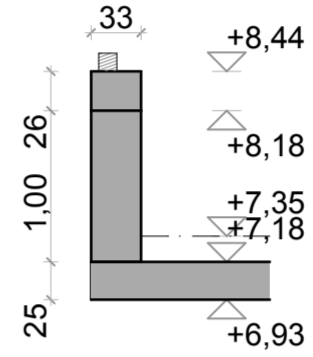
Tp2 TÉRDFALPILLÉR NÉZETE KÉSZÜL: 2db M=1:50
