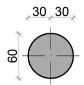
O1 OSZLOP METSZETE KÉSZÜL: 2db M=1:50
