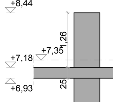
O3 OSZLOP NÉZETE KÉSZÜL: 2db M=1:50
