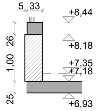
K5 KOSZRÚ METSZETE KÉSZÜL: 2db*9,88fm M=1:50
